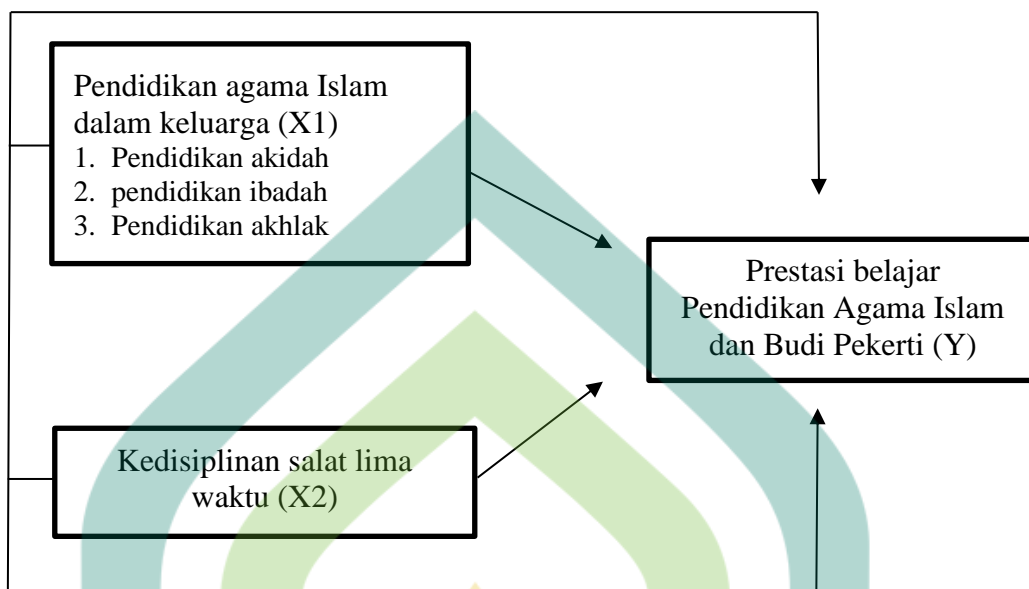
Gambar 1. 1 Kerangka Berpikir
